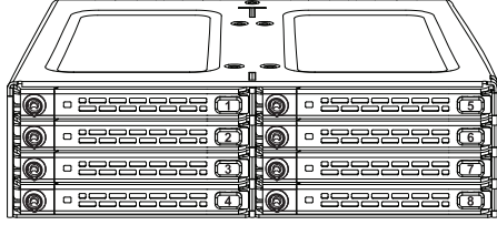
MB998SK-B
